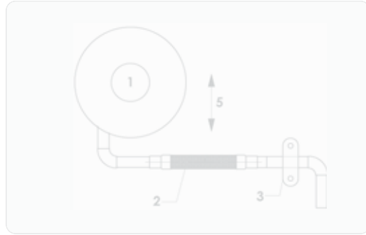
РИС.1 СИСТЕМА С ОДНИМ ВИБРОИЗОЛЯТОРОМ
