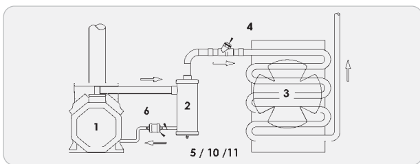
ОДНО КОМПРЕССОРНАЯ СИСТЕМА
